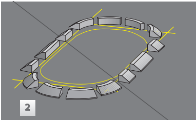
Bereitstellen der Klebebordsteine in der exakten Reihenfolge
