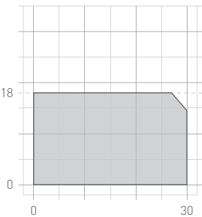
1 – Breitbord mit Absenker auf Pflasterstein 30 x 30 cm, basalt-anthrazit 2 – Breitbord, granit-braun
